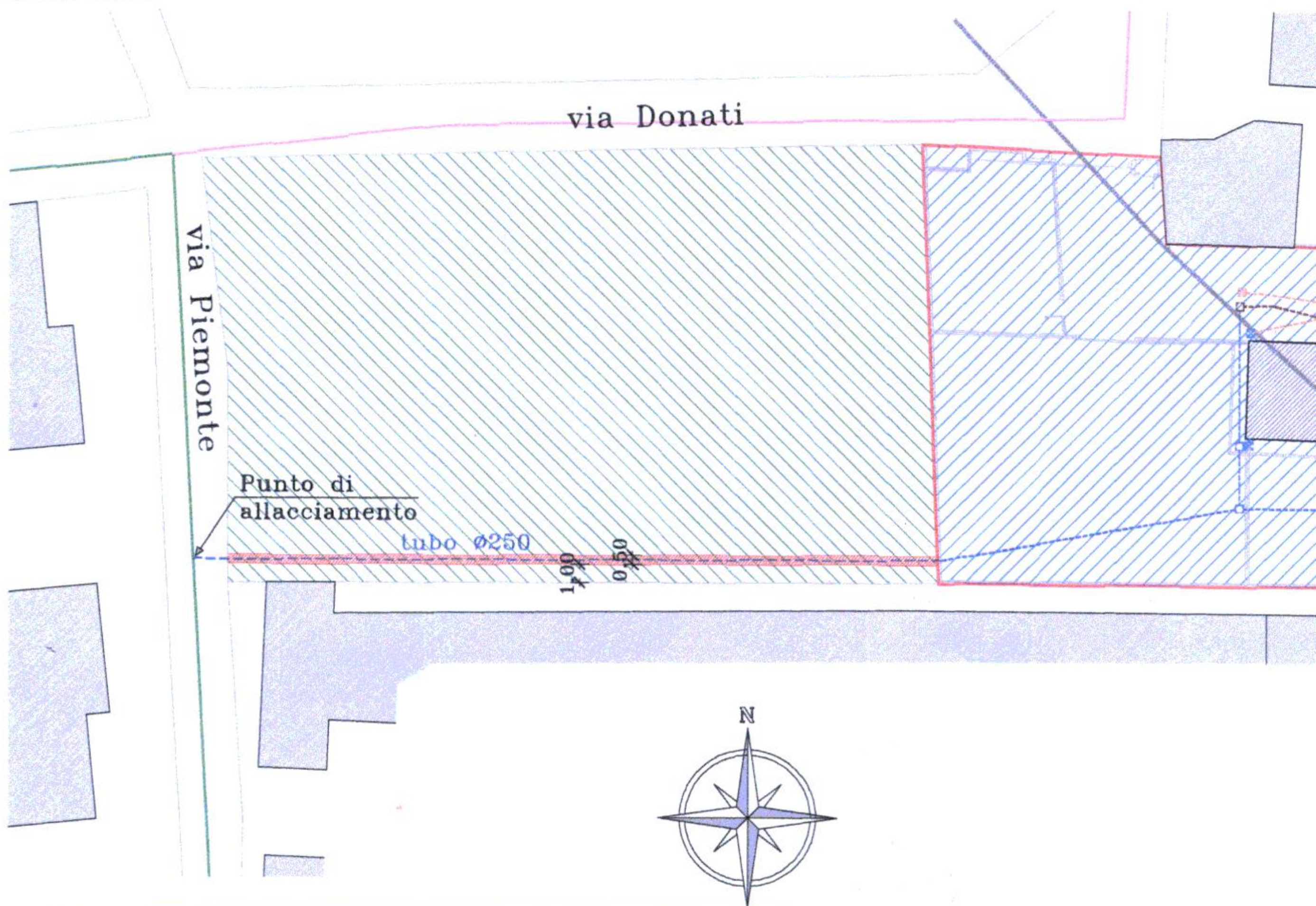
Planimetria lotto e reti scala 1:400
